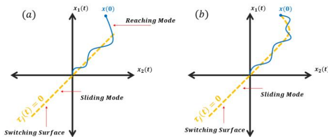
شکل ۲: مفهوم کنترل حالت لغزشی: (a) کنترل حالت لغزشی معمولی. (b) کنترل حالت لغزشی سراسری.
