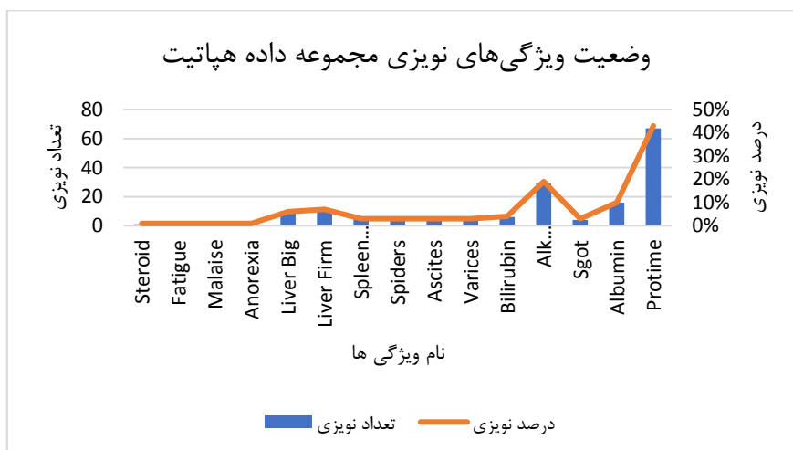
شکل ۴: وضعیت ویژگی‌های نویزی مجموعه داده هپاتیت C
