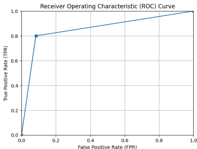
شکل ۲: نمودار ROC
