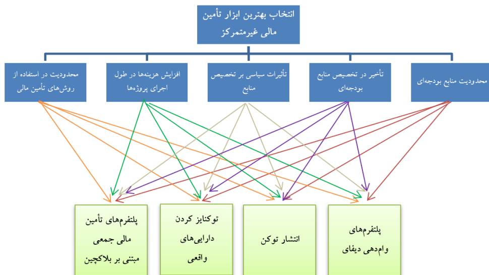
شکل شماره (۲) تحلیل سلسله‌مراتبی تصمیم‌گیری چند معیاره در پژوهش حاضر منبع: یافته‌های پژوهش
