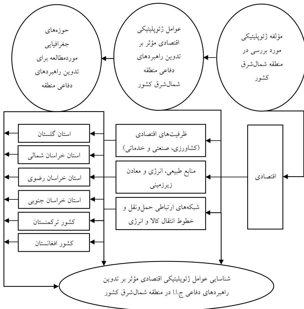
شکل ۱: چارچوب نظری
