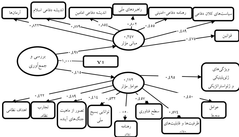
شکل ۱۰: مدل‌سازی معادلات ساختاری بُعد «بررسی و جمع‌آوری اطلاعات» و عوامل و زیر عامل‌های آن
