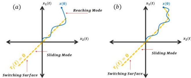
شکل ۲: مفهوم کنترل حالت لغزشی: (a) کنترل حالت لغزشی معمولی. (b) کنترل حالت لغزشی سراسری.
