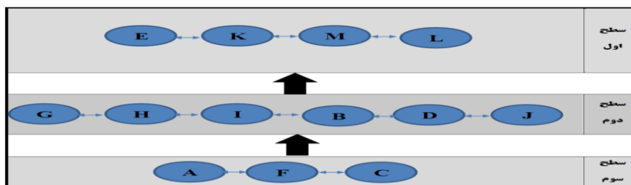
مدل شماره (۱): مدل ساختاری - تفسیری تحقیق حاضر
