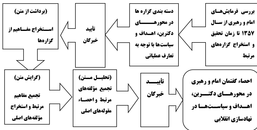
شکل ۳: الگوی مراحل مختلف تحلیل گفتمان امام و رهبری
