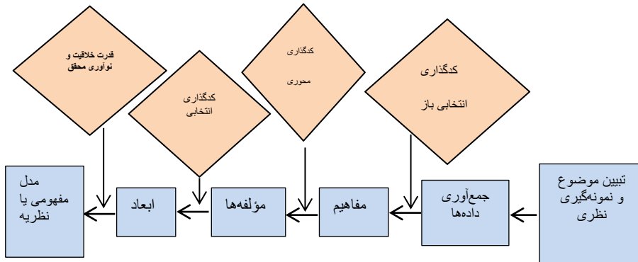
شکل ۲: مدل توسعه یافته فرایند اجرای گراند تئوری (زارعی، ۱۳۸۷: ۹۸)
